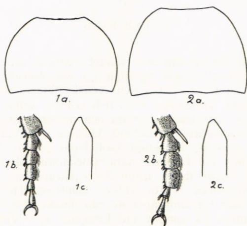
1. Oodes gracilis Villa. — 2. O. helopioides Fbr. — a. Halsskölden. — b. Högra framtarsen hos ♂. — c. Penisspetsen ovanifrån. (Auctor del.).
